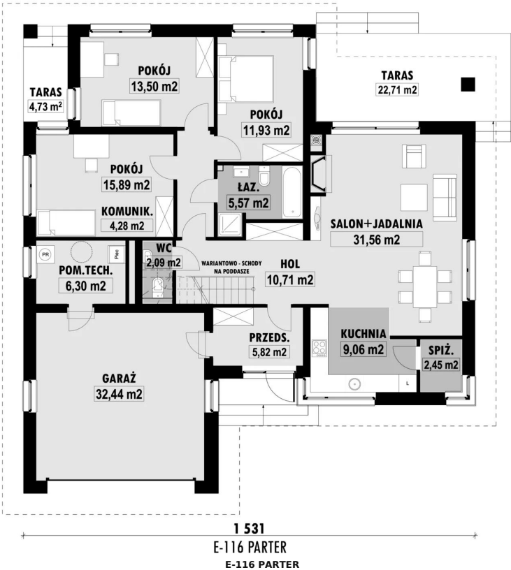
RZUT PARTERU
