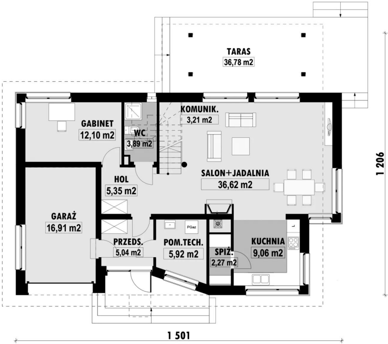
RZUT PARTERU
