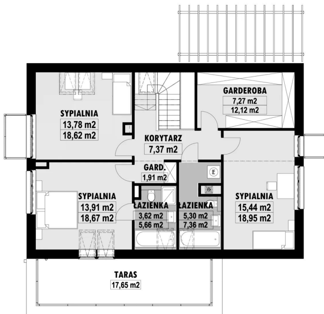
E-102 PODDASZE E-102 PODDASZE
