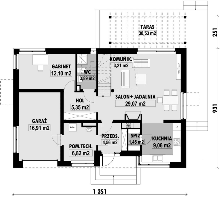
RZUT PARTERU
