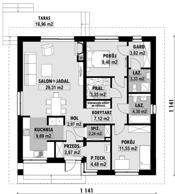
E-271-L PARTER E-271 PODDASZE - OPCJA
