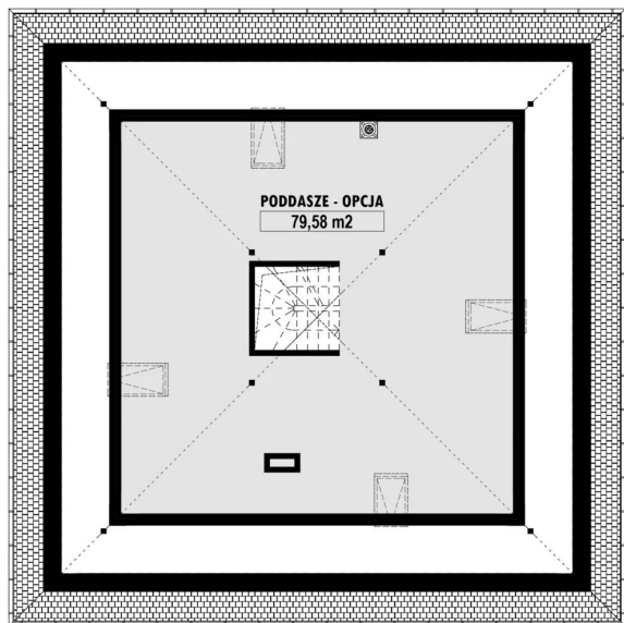
E-269 PODDASZE E-269 PODDASZE - OPCJA
