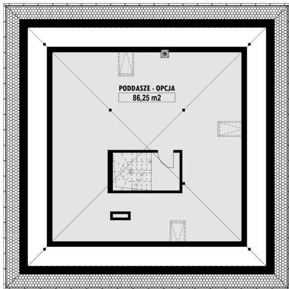
E-268 PODDASZE E-268 PODDASZE - OPCJA
