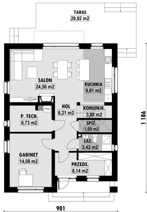
✕ RZUT PARTERU
