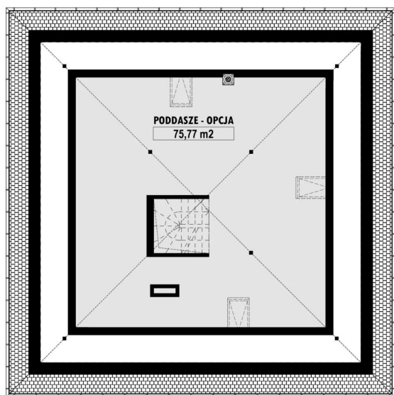
E-266a PODDASZE E-266 PODDASZE - OPCJA
